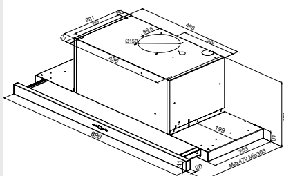
Montageabstand über Kochfeld Elektro 550 mm, Gas 650 mm
