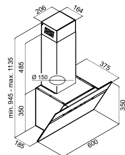
Montageabstand über Kochfeld Elektro 450 mm, Gas 650 mm
