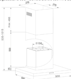
Montageabstand über Kochfeld Elektro 650 mm, Gas 750 mm
