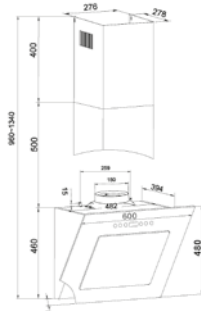
Montageabstand über Kochfeld Elektro 450 mm, Gas 650 mm
