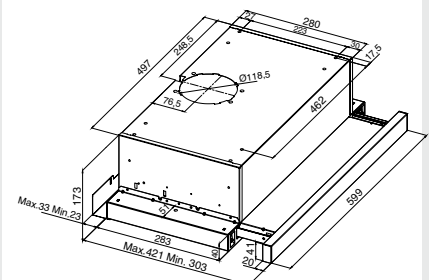
Montageabstand über Kochfeld Elektro 550 mm, Gas 650 mm
