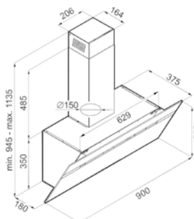
Montageabstand über Kochfeld Elektro 450 mm, Gas 650 mm
