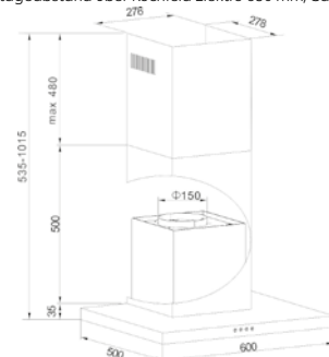
Montageabstand über Kochfeld Elektro 650 mm, Gas 750 mm
