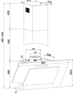
Montageabstand über Kochfeld Elektro 450 mm, Gas 650 mm
