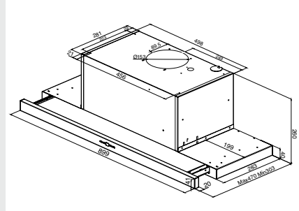
Montageabstand über Kochfeld Elektro 550 mm, Gas 650 mm
