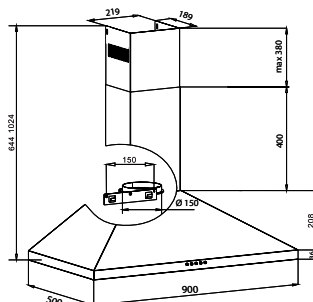
Montageabstand über Kochfeld Elektro 650 mm, Gas 750 mm
